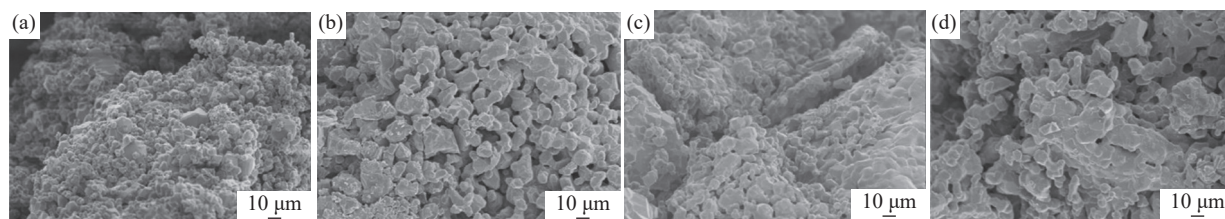
(a) 转炉渣-还原氧化循环 5 次; (b) 电炉渣-还原氧化循环 5 次; (c) 转炉渣-还原氧化循环 10 次; (d) 电炉渣-还原氧化循环 10 次
