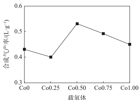
图1 不同掺杂比例 Co 金属改性 Ca 2 Fe 2 O 5 载氧体对合成气产率的影响 [27]
