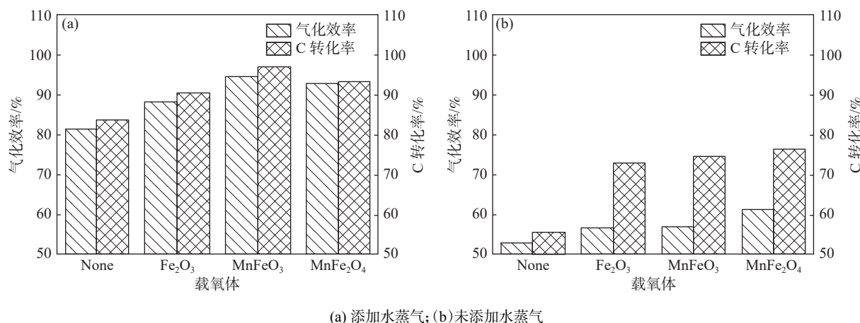
图 2 不同铁基载氧体化学链气化性能参数对比 [29]
