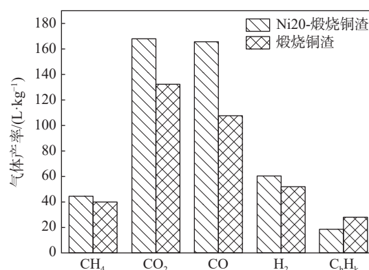
图 4 掺杂 Ni 金属铜渣对合成气组分产率的影响 [45] Fig. 4 Influence of the Ni doped metal copper slag on syngas component yield [45]
