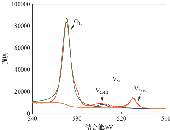
图 3 失活硫酸催化剂 XPS 分析 Fig. 3 XPS spectrum of deactivated sulfuric acid catalyst
