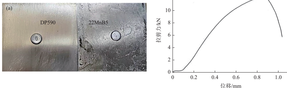
图9 界面断裂的拉伸曲线和断口形貌
