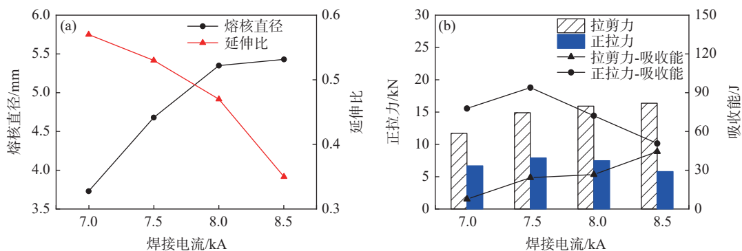
图7 焊接电流对接头拉伸性能的影响
