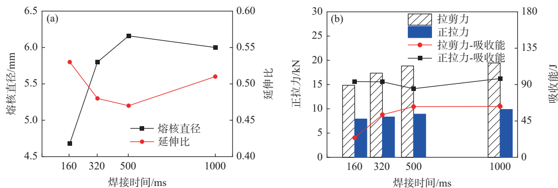
图8 焊接时间对接头拉伸性能的影响
