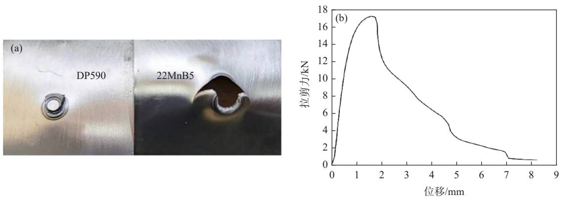
图 10 部分界面断裂的拉伸曲线和断口形貌 Fig. 10 Tensile curves and fracture morphologies of partial interfacial fractures
