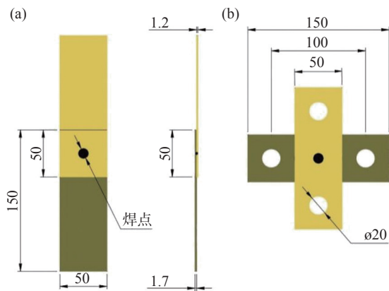
图 1 拉伸试样几何尺寸(单位:mm) Fig. 1 Geometrical parameters of tensile specimens
