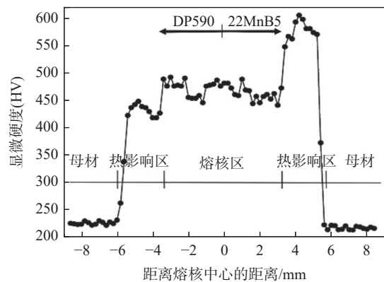
图6 DP590/22MnB5点焊接头显微硬度分布
